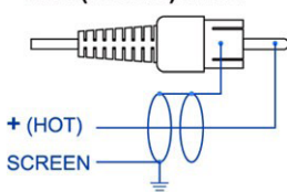
RCA (PHONO) JACK
